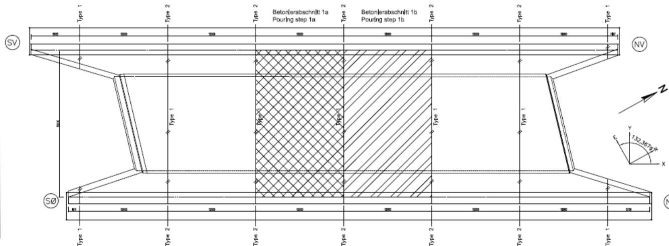
Grundriss Übersicht / Plan view survey - 1:200
