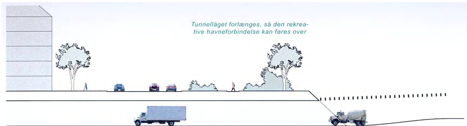
Principielt længdesnit ved tunnelmunding - 1:500
